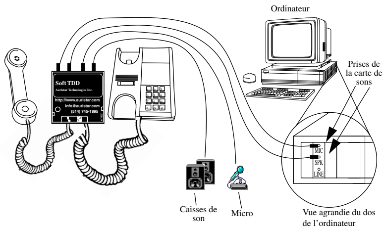
Branchement du module téléphonique
